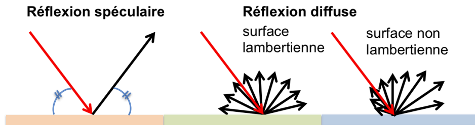
FIGURE 4.2 – Schémas de différents types de réflexion. Le mode varie selon la surface qui reçoit le rayonnement incident, dont la direction est représentée par la flèche rouge ; les flèches noires illustrent les directions d'émergence.
