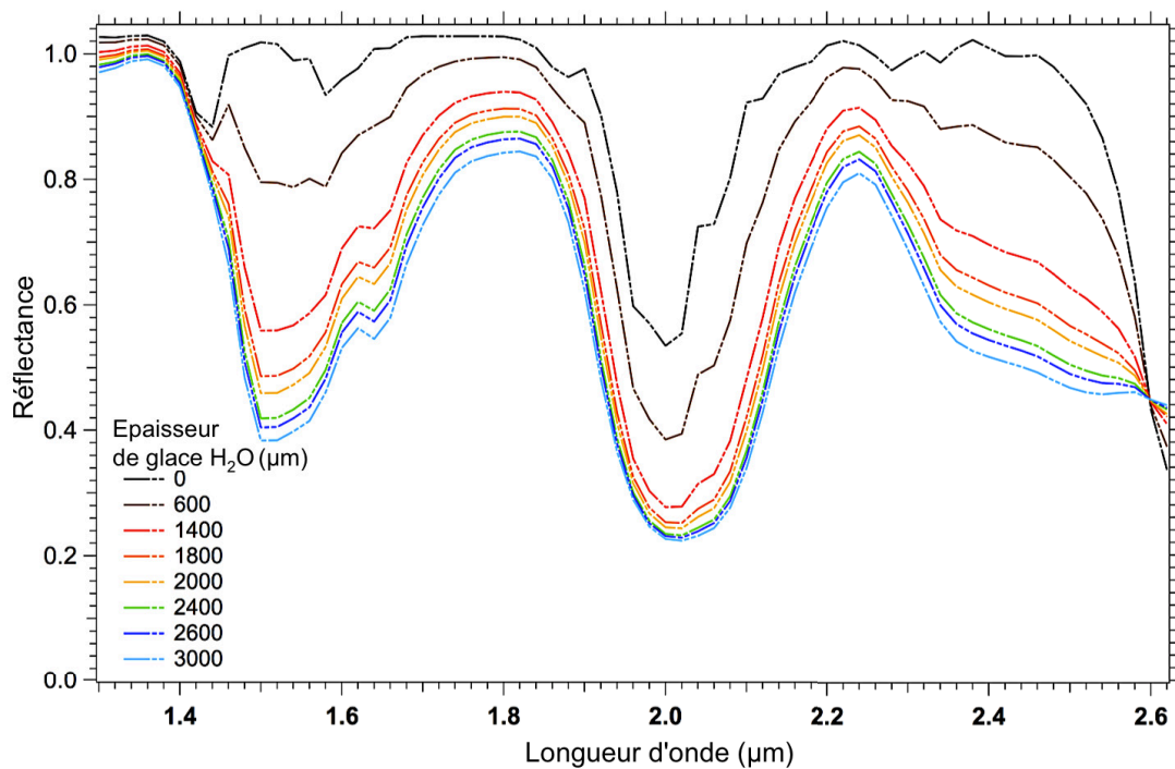
FIGURE 4.17 – Modélisation des spectres de la Figure 4.16. Paramètres utilisés : couche de neige d'eau sur une couche de neige carbonique; grains de 350 \mu\text{m} pour \text{CO}_2 et 40 \mu\text{m} pour \text{H}_2\text{O} ; compacité 50% pour \text{CO}_2 et 10% pour \text{H}_2\text{O} ; les épaisseurs de la couche de \text{H}_2\text{O} associées à chaque courbe sont indiquées en légende sur le graphique.
