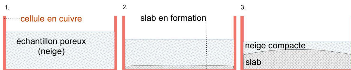
FIGURE 6.5 – Schéma de formation et progression d'un slab à partir de neige compacte par réchauffement de la base, tel qu'observé dans la cellule environnementale de CarboNIR. 1 : Echantillon initial de neige compacte, 2 : Apparition d'un slab au bas de l'échantillon, 3 : Progression du slab à l'intérieur de l'échantillon.
