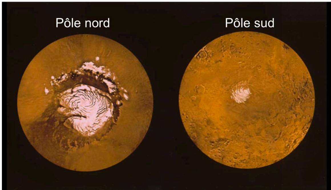
FIGURE 1.2 – Vue des calottes polaires permantes de Mars, nord à gauche (1000 km de diamètre), sud à droite (calotte résiduelle sur 300 km de diamètre). Montage d’images NASA/Viking.
