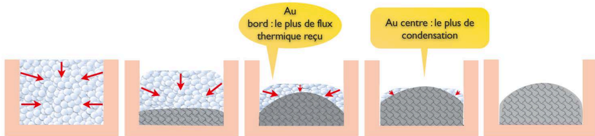
FIGURE 6.14 – Schéma des flux thermiques incidents dans la neige à l'origine de la progression du slab.
